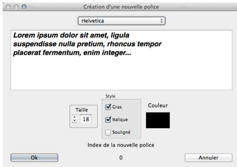
FIGURE 10 – Dialogue de création des polices
