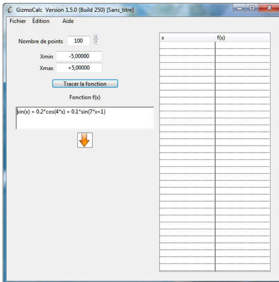
FIGURE 3 – Fenêtre principale. À gauche on a la définition des paramètres de l'application : le nombre de points N , l'intervalle de définition (X_{\min}, X_{\max}) et la définition de la fonction. À droite on a l'emplacement de la table (x, f(x)) où seront reportées les valeurs du calcul. À noter que les labels Xmin et Xmax disposent de menus contextuels (accessibles par un click droit) permettant de simplifier l'entrée des données. En cliquant sur le bouton Tracer la fonction , le calcul est lancé. Les résultats apparaissent sur la figure [4].
