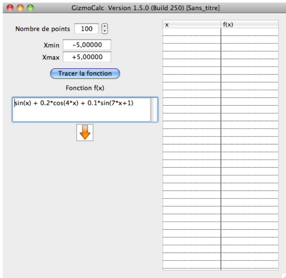
FIGURE 3 – Fenêtre principale. À gauche on a la définition des paramètres de l'application : le nombre de points N , l'intervalle de définition (Xmin, Xmax) et la définition de la fonction. À droite on a l'emplacement de la table (x, f(x)) où seront reportées les valeurs du calcul. À noter que les labels Xmin et Xmax disposent de menus contextuels (accessibles par un click droit) permettant de simplifier l'entrée des données. En cliquant sur le bouton Tracer la fonction , le calcul est lancé. Les résultats apparaissent sur la figure [4].
