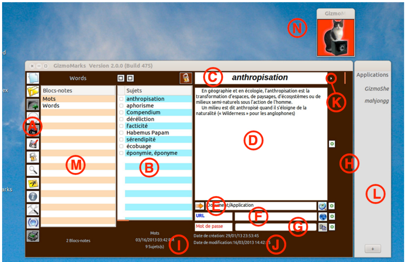
FIGURE 2 – Vue générale de de la fenêtre de l'application. On aperçoit à gauche la liste des blocs-notes ( M ) pour une collection de blocs-notes donnée (ici Mots/Words ) et la liste des sujets ( B ) relative à un bloc-note ( Mots ). Le tiroir des applications fréquentes (à droite) est déployé et le sticker flottant est visible en haut à droite.
