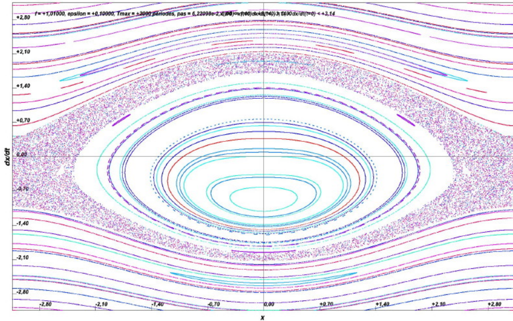
FIGURE 7 – Exemple de balayage automatique : Trajectoires dans l'espace des phases (x, \dot{x}) pour x_i(t = 0) = x_{min} + i\delta x , v_j = \dot{x}_j(t = 0) = v_{min} + j\delta v , \delta x = (\delta x_{max} - \delta x_{min})/N_e , \delta v = (\delta v_{max} - \delta v_{min})/N_e pour 0 \leq i \leq N_e - 1, 0 \leq j \leq N_e - 1 . Avec f = 1,01 , \epsilon = 0,1 , pas constant h = (2\pi/f)/100 , durée du calcul 2000 périodes. Chaque nœud du maillage rectangulaire donne la position des conditions initiales.
